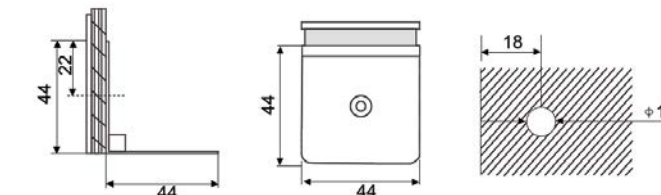
Spojnica kutna zid- staklo 90° inox MAT / inox SJAJ debljina stakla 8/10 mm
