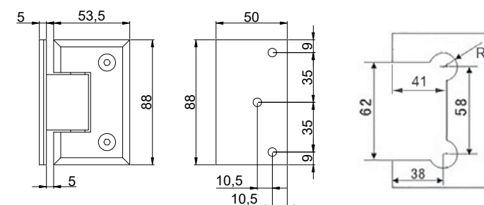
Automatska spojnica* zid-staklo zamaknuta pločica
