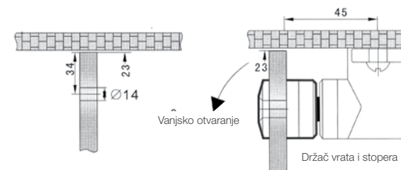
Magnetni stoper debljina stakla 8/10 mm SA 8500E-10 inox MAT
