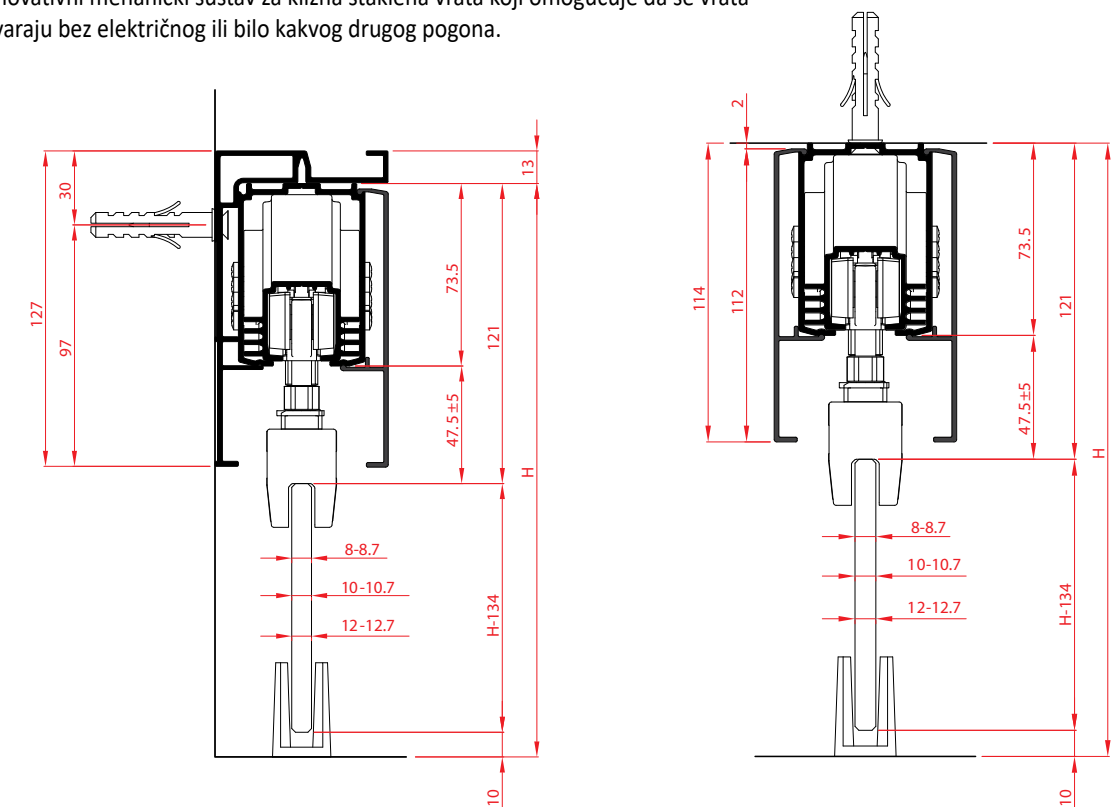
Zidni nosač prihvata vodilice
