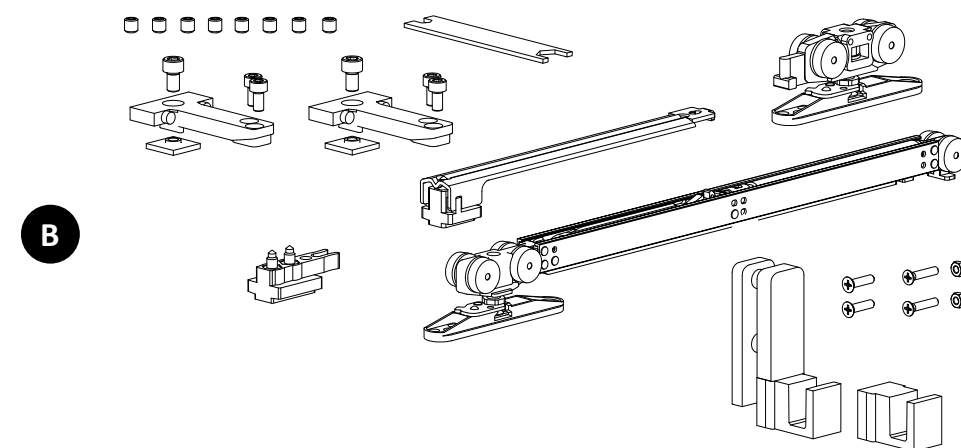
set za srednje krilo V 0342.5
