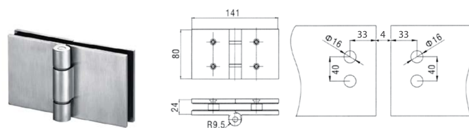
Preklopna spojnica staklo-staklo preklopna
