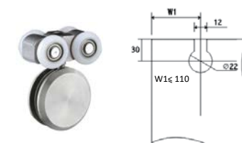
Nosač stakla
