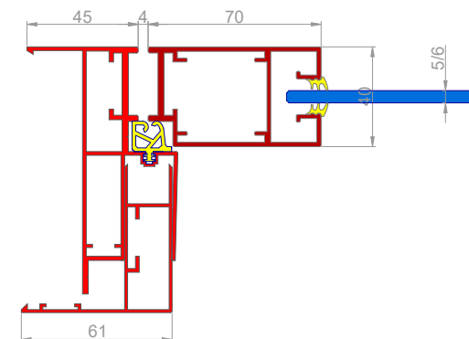
Alu dovratnik OBUHVATNI + ALU profil IG AO
