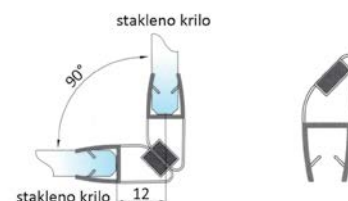
Magnetna brtva 90° 2500 mm prozirna TA PS-10M/6 (za staklo 6 mm) prozirna / crna TA PS-10M/8 (za staklo 8 mm) prozirna TA PS-10M/10 (za staklo 10 mm)
