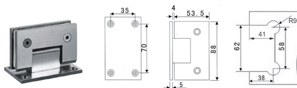
Automatska spojnica zid-staklo 90°
