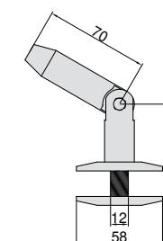
Konektor za nadstrešnicu staklo-šipka
