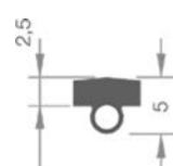
Guma za staklo debljina stakla 6 mm
