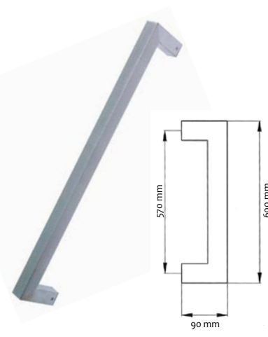
Rukohvat dužina 600 mm 30 x 30 mm priprema stakla Ø16 mm u paru
