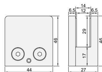
Spojnica zid - staklo inox SJAJ / MAT debljina stakla 10 mm
