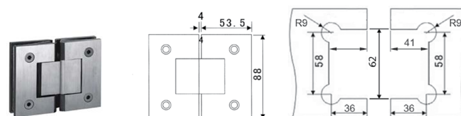
Automatska spojnica staklo-staklo ravna
