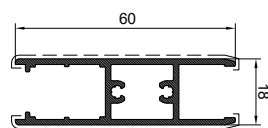
Nosač stakla
