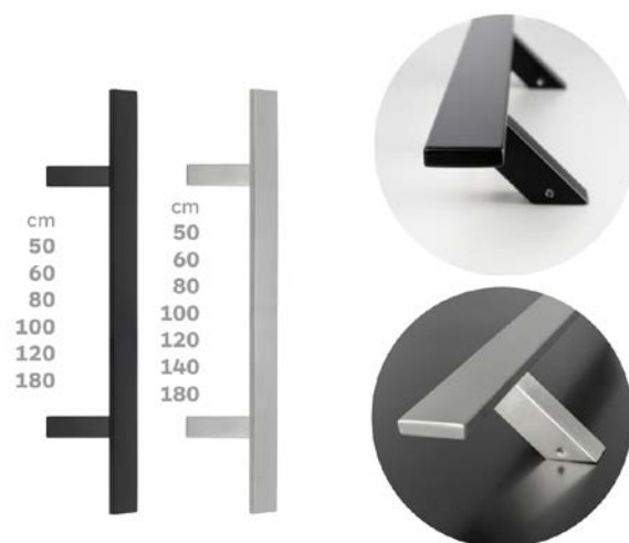
Rukohvat dimenzija 40x10 mm priprema stakla Ø14 mm ID Rukohvat inox 45° kvadratni crni mat / inox 316 SAT
