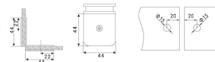
Spojnica kutna 90° inox MAT / inox SJAJ debljina stakla 8/10/12 mm
