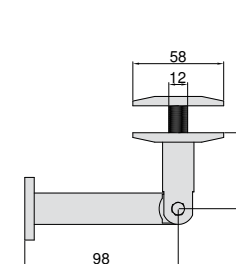
Konektor za nadstrešnicu zid-staklo
