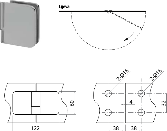
Podizna spojnica staklo-staklo debljina stakla 8/10 mm nosivost 45kg maksimalan krak 750 mm lijeva / desna
