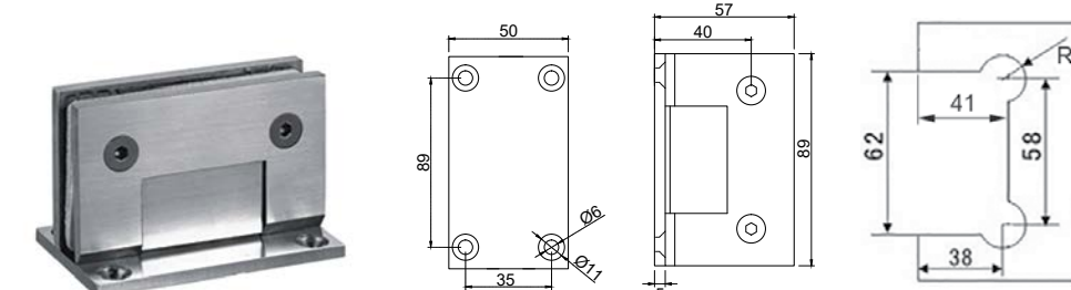
Fiksna spojnica zid-staklo
