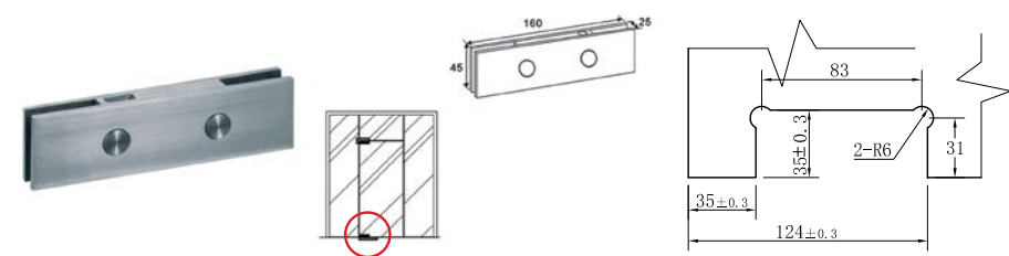
Spojnica donja SA 7101
