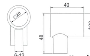
Konektor* okretni staklo-šipka debljina stakla 6/12 mm SA 8500E-14 inox / crno
