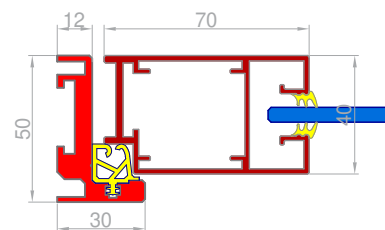
Alu dovratnik IG AD 5700 "L" + ALU profil IG AO
