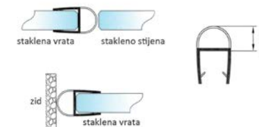
Brtva s polukružnim završetkom 2500 mm prozirna TA PS-11/6 (za staklo 6 mm) prozirna / crna TA PS-11/8 (za staklo 8 mm) prozirna TA PS-11/10 (za staklo 10 mm)
