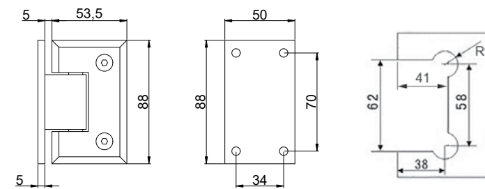
Automatska spojnica* zid-staklo 90°
