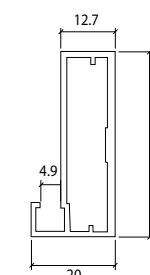
Alu profil za staklo debljina stakla 4 mm
