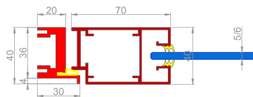
Alu dovratnik "INVISIBLE EVOLUTION" + ALU profil IG AO
