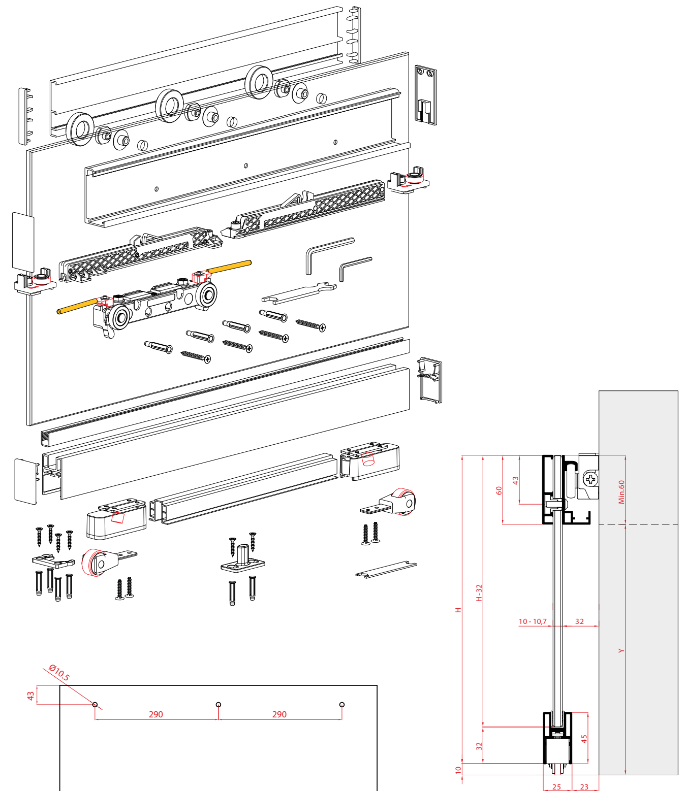
V Magic 2 Set za STAKLO
