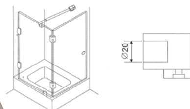
Konektor* okretni zid-šipka SA 8500E-15 inox / crno
