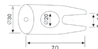
Konektor* fiksni staklo-šipka debljina stakla 6/12 mm SA 8500E-12 inox / crno
