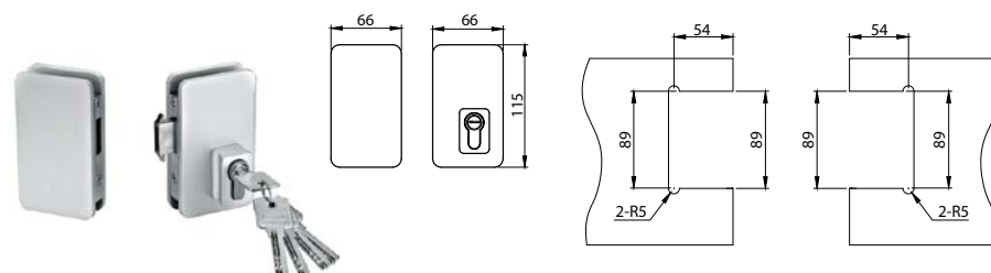
Brava za klizna vrata s cilindrom* aluminij
