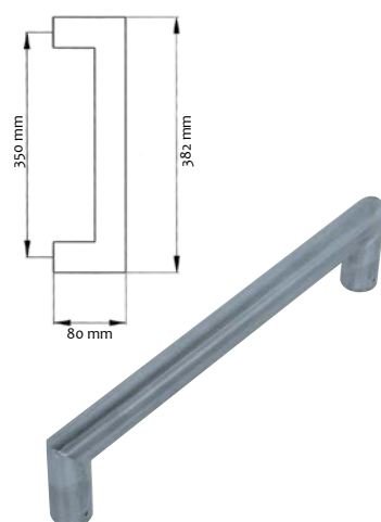
Rukohvat dužina 382 mm promjer Ø32 priprema stakla Ø16 mm u paru
