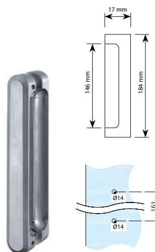
Ručkica za klizna vrata razmak 161 mm priprema stakla Ø14 mm u paru
