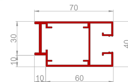
IG AO Aluminijski okvir
