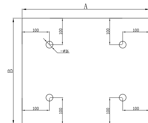
INOX 304 / INOX 316 Colni navoj!
