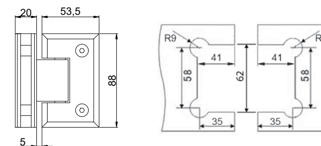
Automatska spojnica* staklo-staklo 90°
