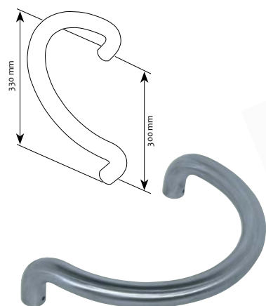
Rukohvat dužina 330 mm promjer Ø32 priprema stakla Ø16 mm u paru
