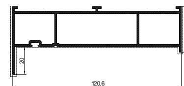
Bočni profil 5 krila
