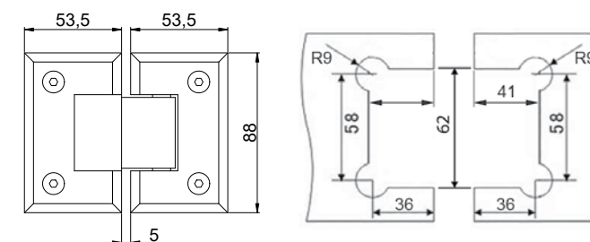
Automatska spojnica* staklo-staklo ravna
