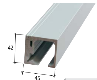
Aluminijska vodilica 1X
