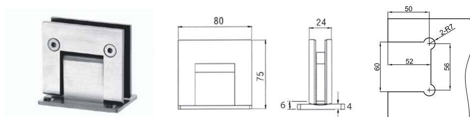
Okretna spojnica zid-staklo
