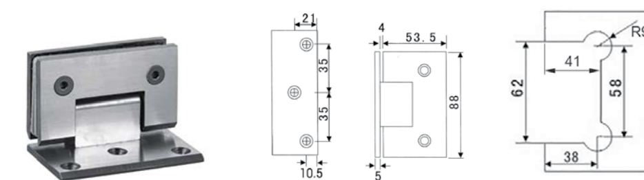
Automatska spojnica zid-staklo zamaknuta pločica
