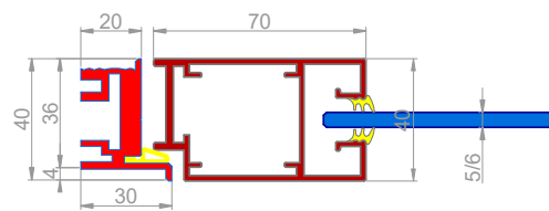
Alu dovratnik "INVISIBLE" + ALU profil IG AO
