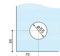
Brava podna s cilindrom i prihvatnikom 70x115 mm, inox MAT SA 7060
