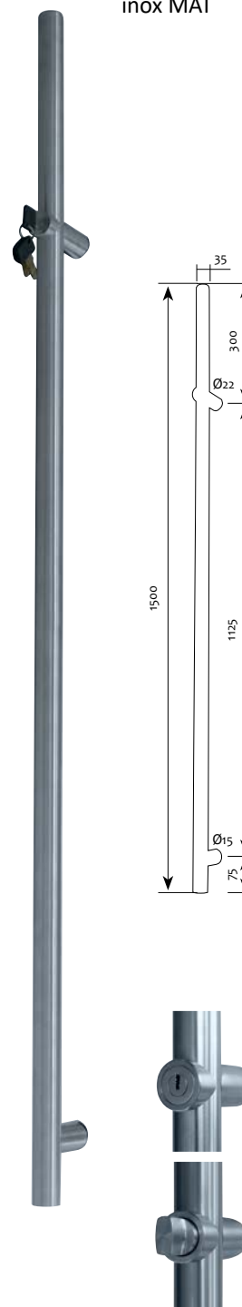
Rukohvat s cilindrom dužina 1500 mm Ø 35 mm ključ / gumb u paru
