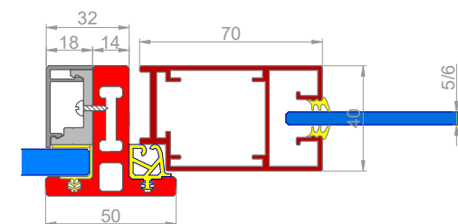
Alu dovratnik IG AD 5700 "T" + ALU profil IG AO
