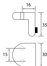
Provodnik debljina stakla 8/10/12 mm SA 8300A-5A inox SJAJ / inox MAT
