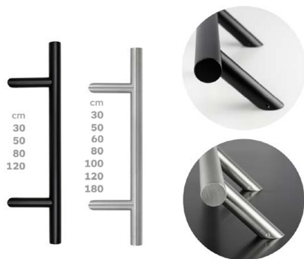
Rukohvat promjer Ø20 priprema stakla Ø14 mm ID Rukohvat inox 45° okrugli crni mat / inox 316 SAT
