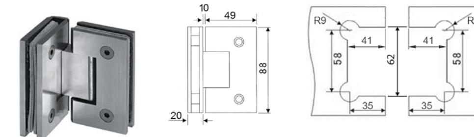
Automatska spojnica staklo-staklo 90°
