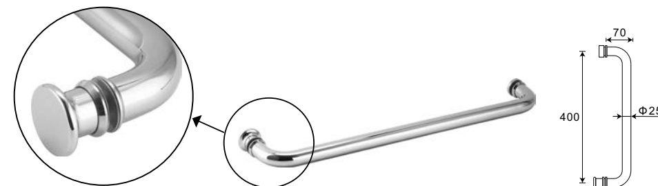
Držac ručnika - ručica za tuš kabinu Ø 25 mm priprema stakla Ø 10 mm
